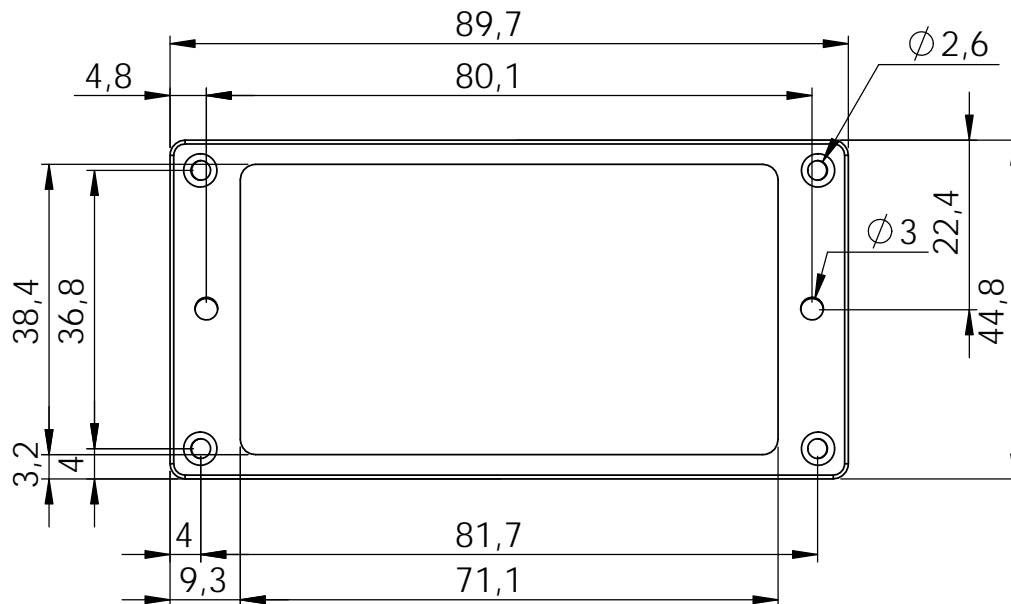
Draufsicht top view
