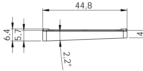
Seitenansicht von links side view left
